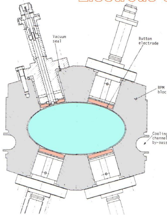
Bloc BPM typique pour machine
