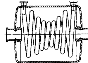
Résonateur à « hélice effilée » 81 MHz - \beta=0,09 (KFK → Saclay)
