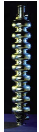
Cavité TTF 1,3 GHz - \beta = 1
