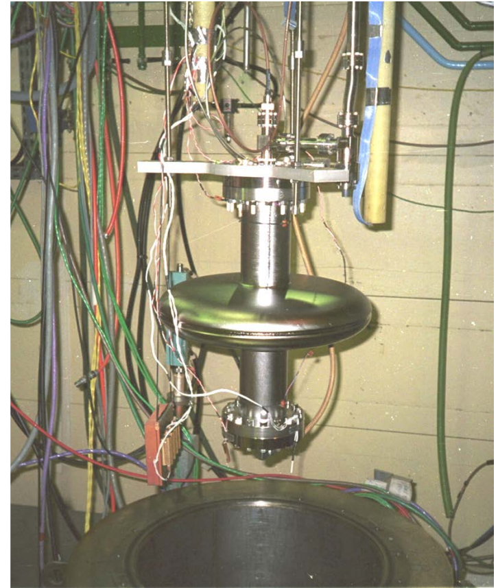
Cavité 700 MHz sur son insert avant encuvage
