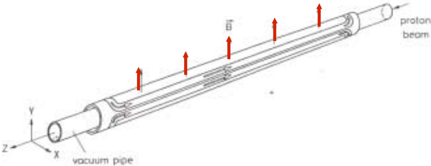
Dipôle 2 en 1 LHC
