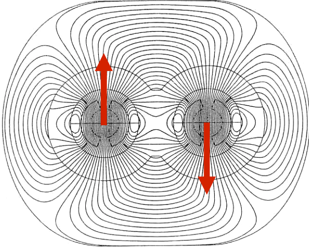
Dipôle 2 en 1 LHC
