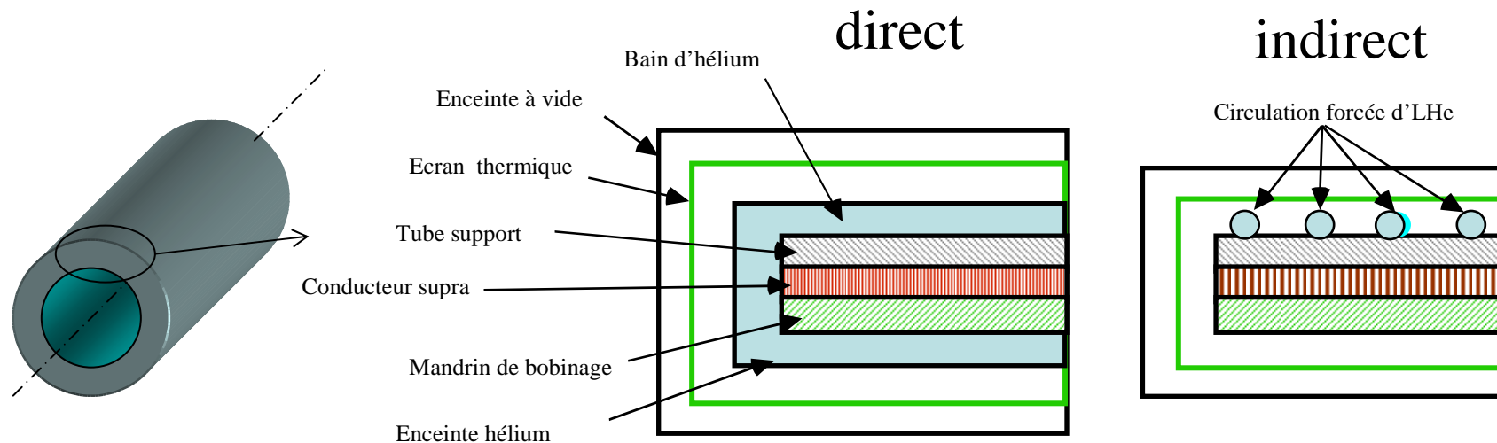
Exemple sur la coupe d'un aimant solénoïde
