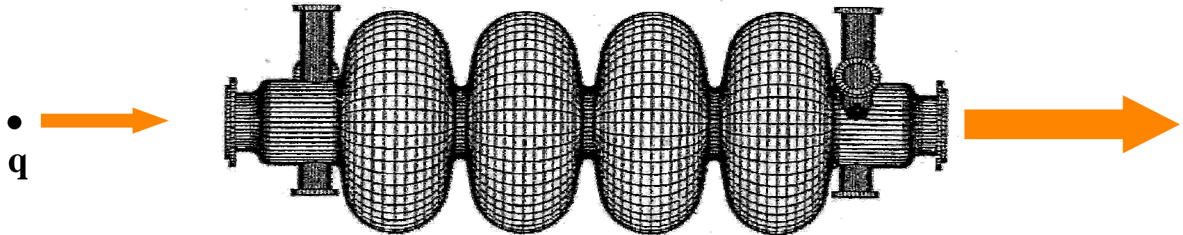
Cavité 4 cellules
