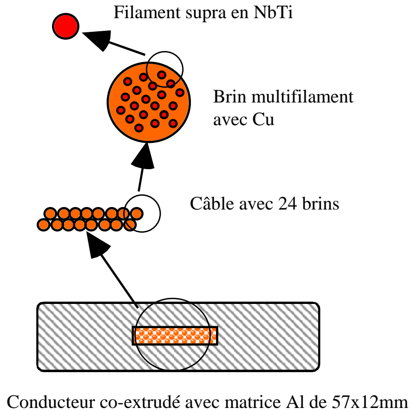
Conducteur ATLAS toroïde (T=4.2 ,K)
